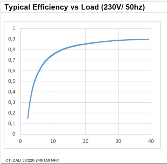
OTi DALI 35220-2401A0 NFC
